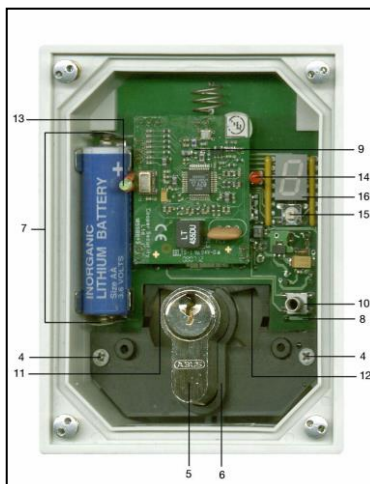
Afb. 2 Behuizing open (met printplaat)
